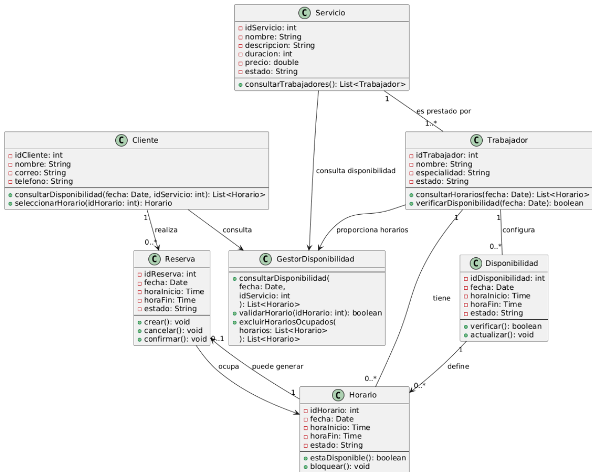
Diagrama de Clases - Visualizar Horarios de Trabajadores Disponibles
